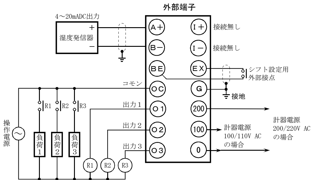
■ R1, R2, R3は補助リレーです。負荷に1 A以上流れる場合は図の様に補助リレーを介して負荷の開閉を行って下さい。
